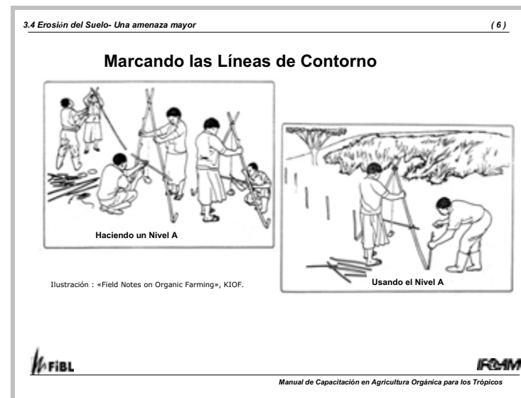
Transparencia 3.4.3(6): Construyendo y usando un Nivel A para identificar las curvas de nivel. Fuente: "Field Notes on Organic Farming", KIOF).
